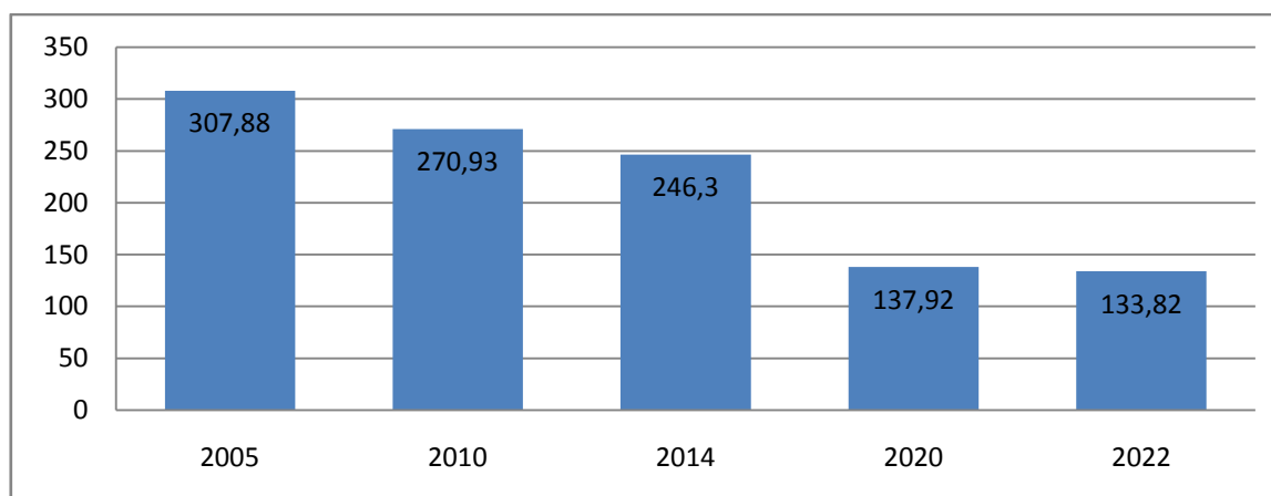
Wykres. Emisja CO 2 [Mg CO 2 /rok] na terenie Gminy Stromiec na potrzeby oświetlenia ulicznego wraz z prognozą na rok 2022. 89
